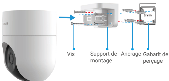
Fig. 2 Montage mural
